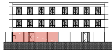
NOORDWESTGEVEL (binnenplein)
